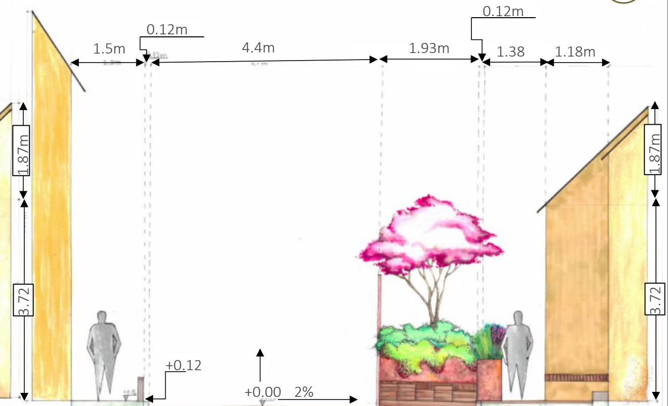
PROFIL TRANSVERSAL - SITUAȚIA PROPUȘĂ
