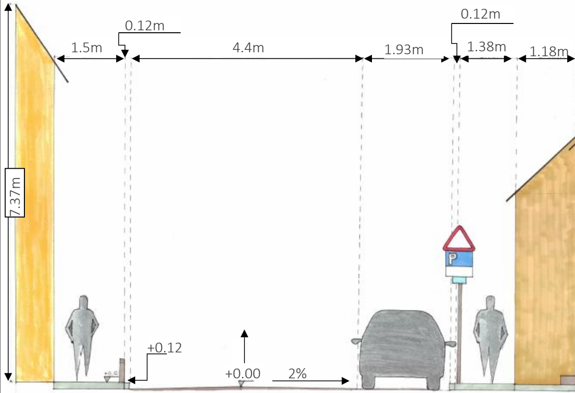
PROFIL TRANSVERSAL - SITUAȚIA EXISTENTĂ
